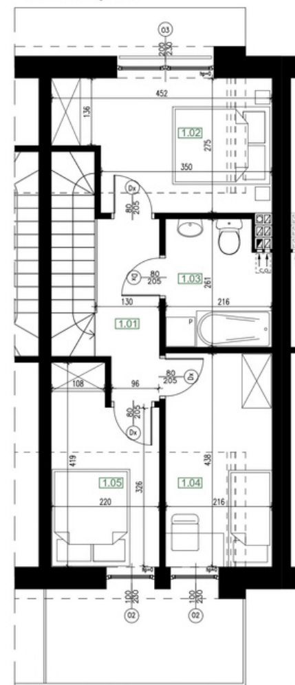
RZUT PIĘTRA
