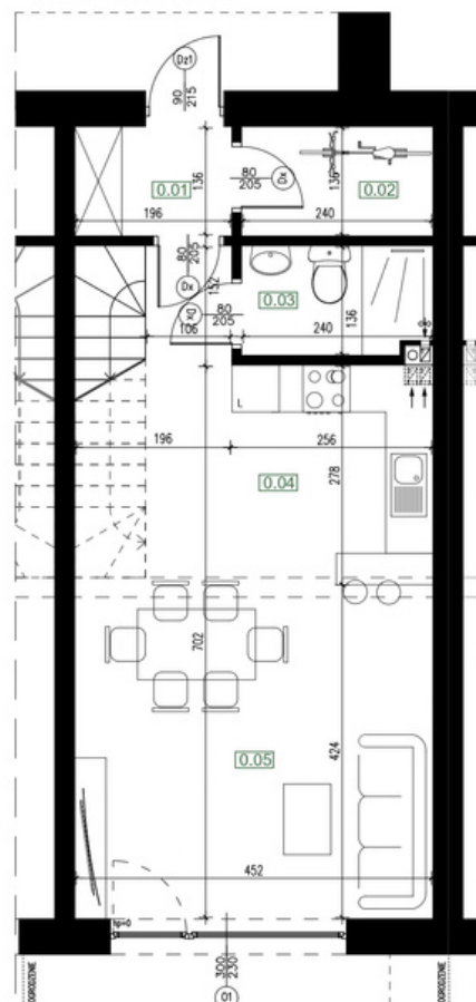
RZUT PARTERU
